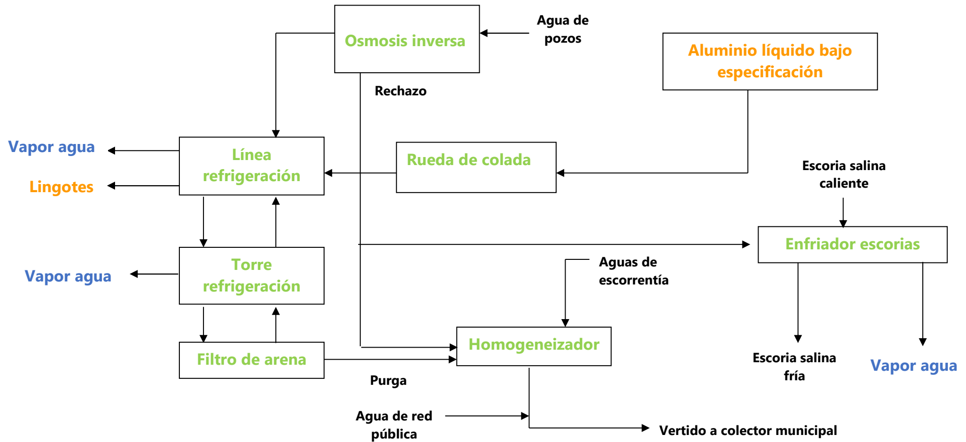
Imagen 4: Diagrama de flujo de proceso para fabricación de lingotes.
